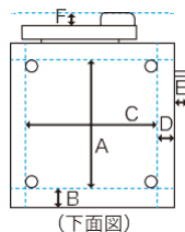
(下面図)
