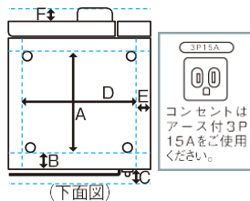
(下面図)
